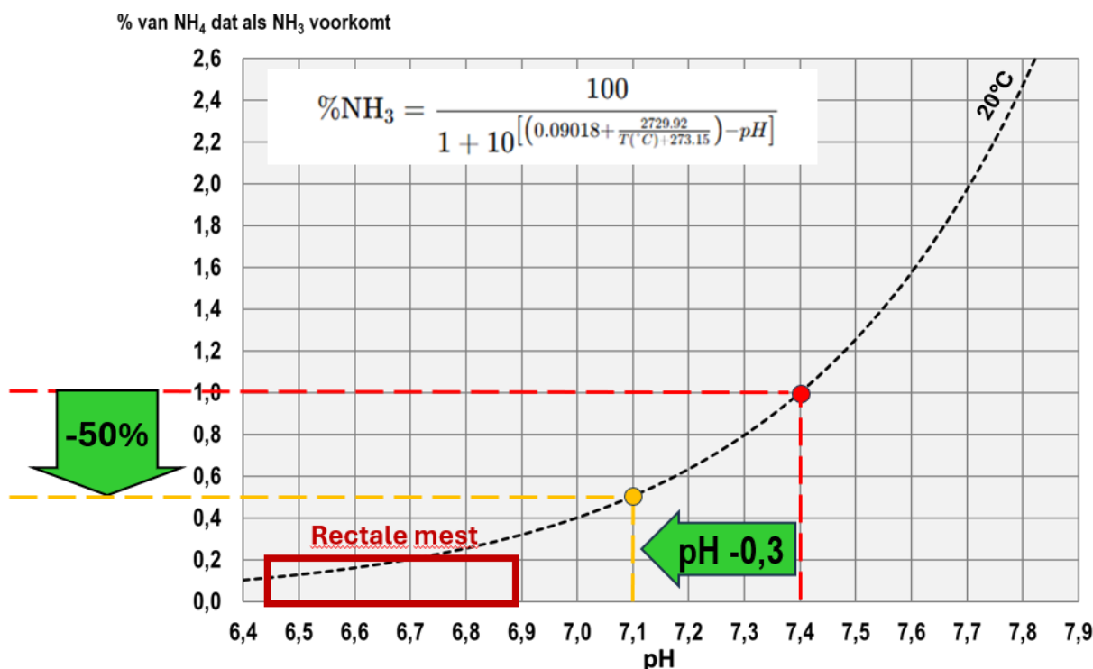
Grafiek 1: Effect van pH op het ammoniak emissie potentieel (AEP)
