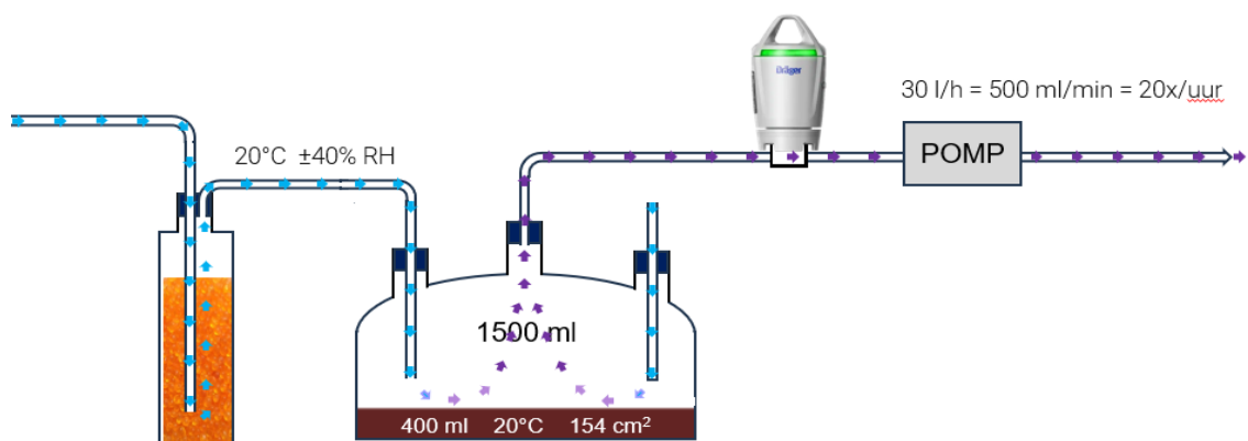
Figuur 2: Proefopstelling voor de AEP-meting.
