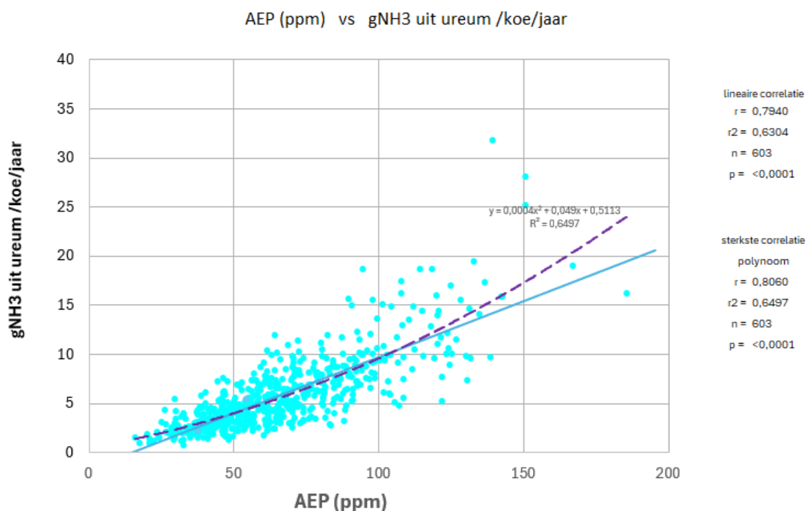
Grafiek 2: Gemeten AEP tegenover het berekende emissiepotentieel vanuit de pH en de ureumvracht (TOPMEST, n = 603 ).
